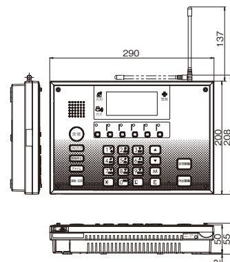
■外形寸法図（単位：mm）
