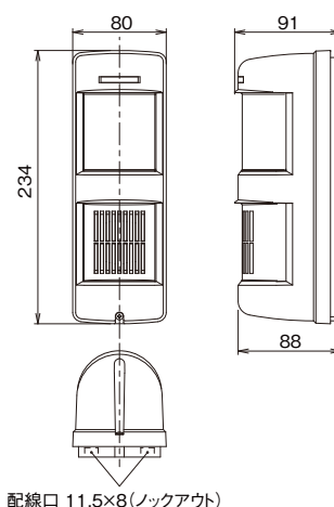
配線口 11.5×8 (ノックアウト)
