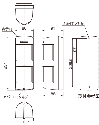
■外形寸法図(単位:mm)
